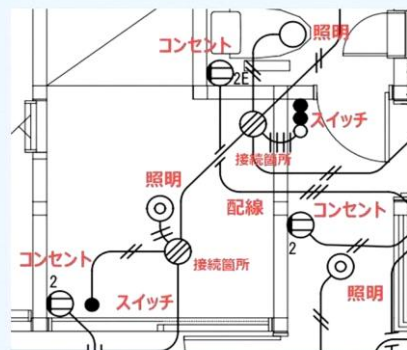
屋内配線図 (例)
