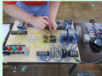
リレーシーケンス制御
